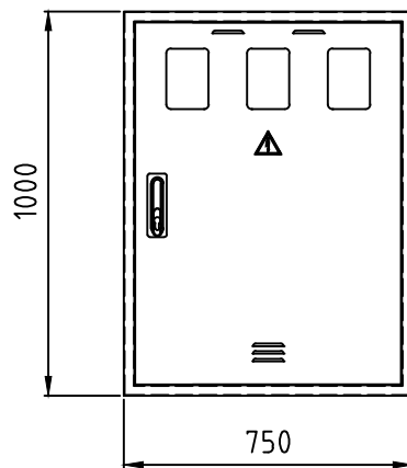
Zunanji izgled omarice:
